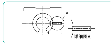
图D-7 销固定
