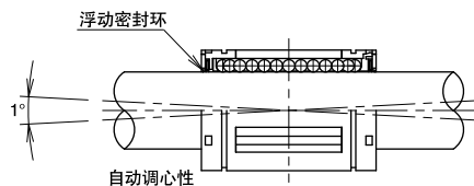
图D-2 浮动密封环及自动调心性
