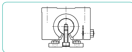
图D-6 开放型
